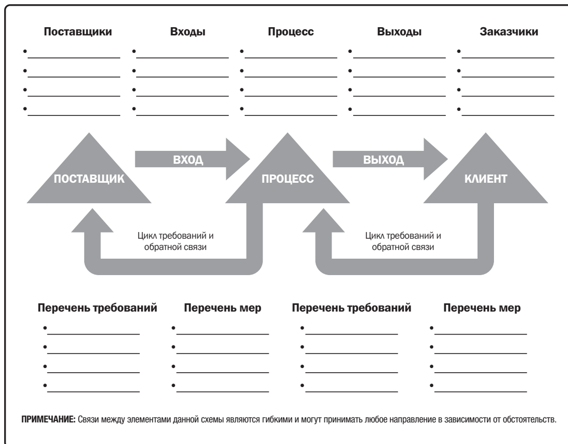
Рис. 8-6. Модель SIPOC
